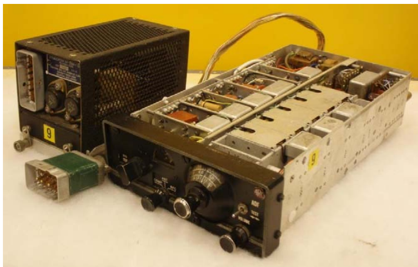
Radiopejl ADF Typ: ARC-318G ( Aircraft Radio Corp )
