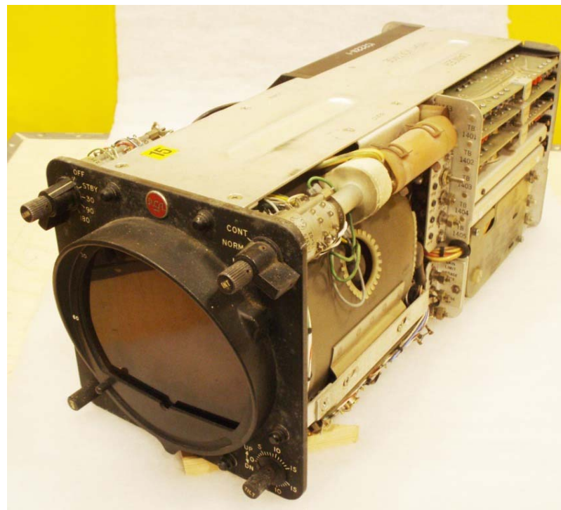
Väderradar Typ RCA AVQ-20
