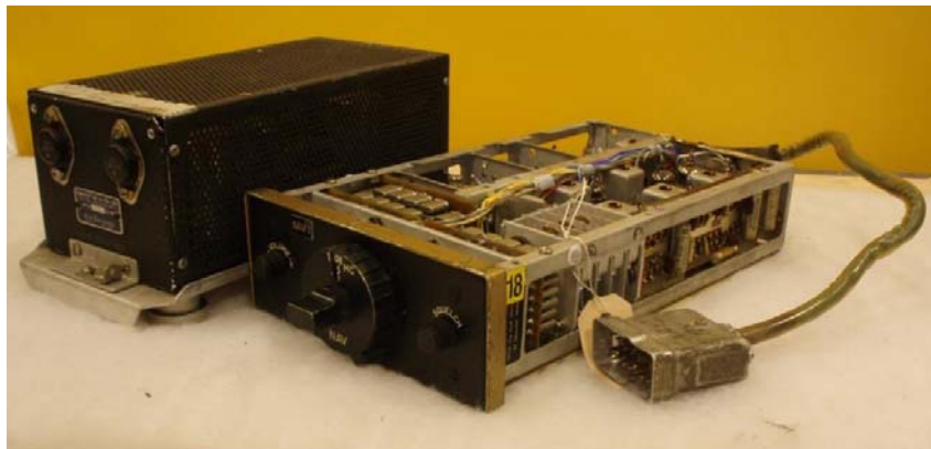
Navigationsradio Cessna -500 Tillverkad av ARC för Cessna 1964. 200 kanaler VOR-LOC-GP.15 radiorör 60 kristaller.Separat kraftomformare . Från:Hallins Flygradio Torslanda/Säve
